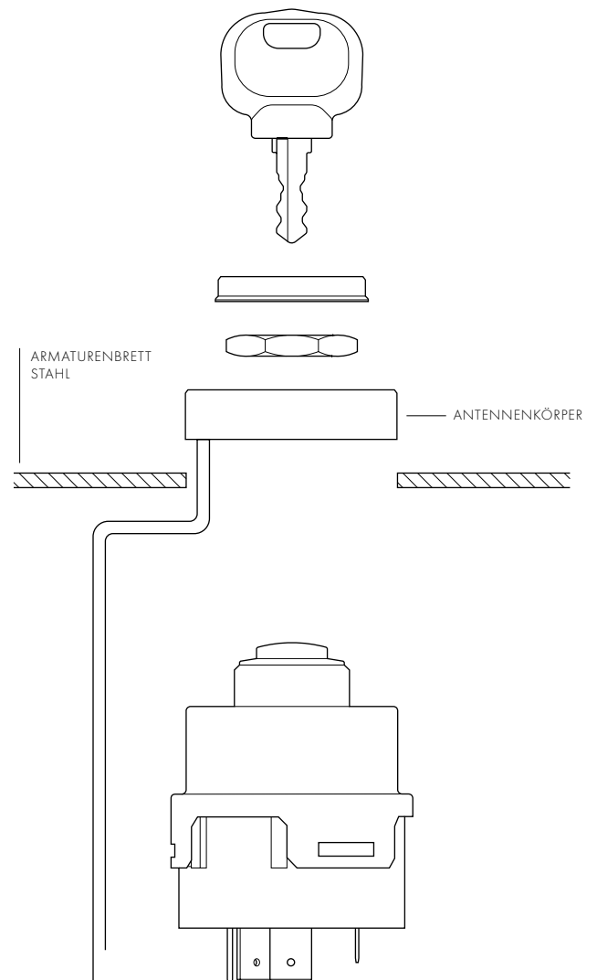
33 99 20 Montage der Antenne oberhalb des Stahl-Armaturenbretts [Faraday-Effekt]
