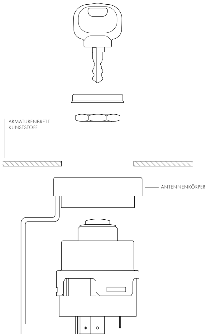
33 99 10 Montage der Antenne unterhalb des Kunststoff-Armaturenbretts
